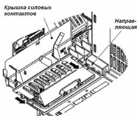
Рисунок 2.6 Установка крышки (для ПЧ мощностью 5.5 и 7.5 кВт)
