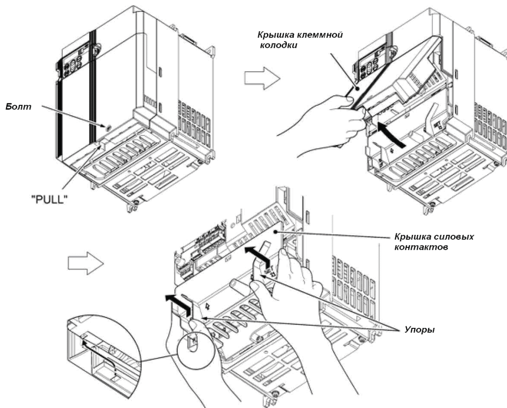
Рисунок 2.5 Снятие крышек (для ПЧ мощностью 5.5 и 7.5 кВт)
