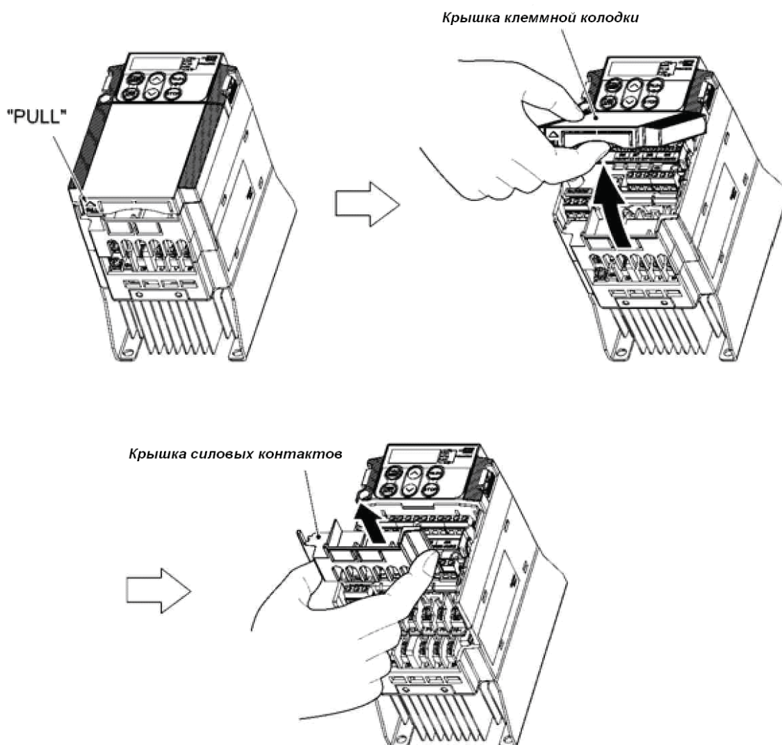
Рисунок 2.4 Снятие крышек
