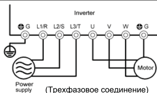
Рисунок 4.1 Соединение контактов цепи питания
