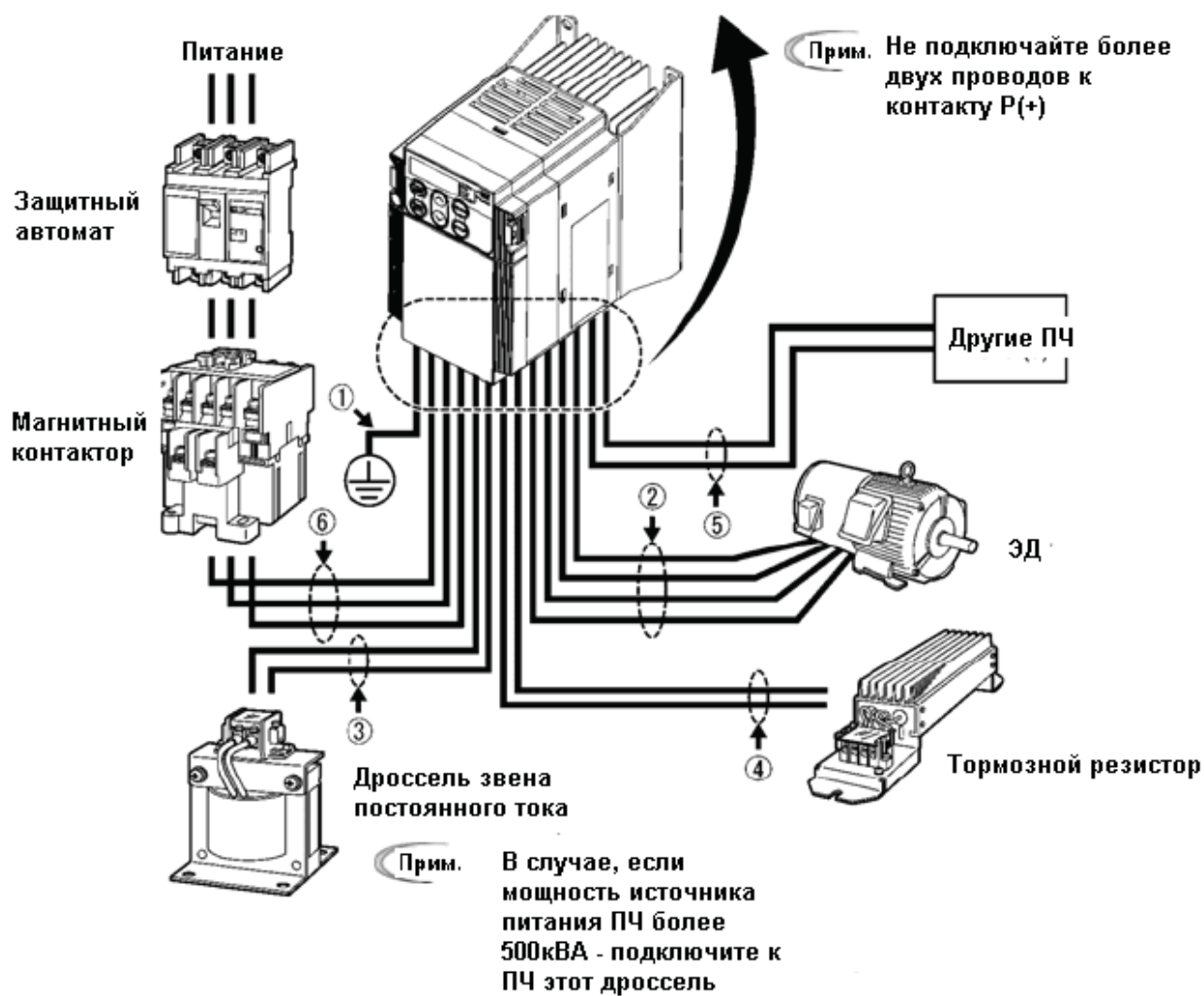
Рисунок 2.9 Подключение к ПЧ периферийного оборудования
