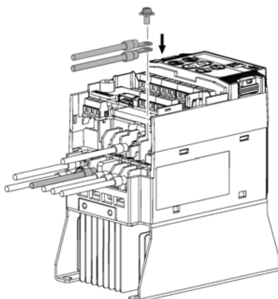
Рисунок 2.11 Подключение тормозного резистора с дросселем звена постоянного тока
