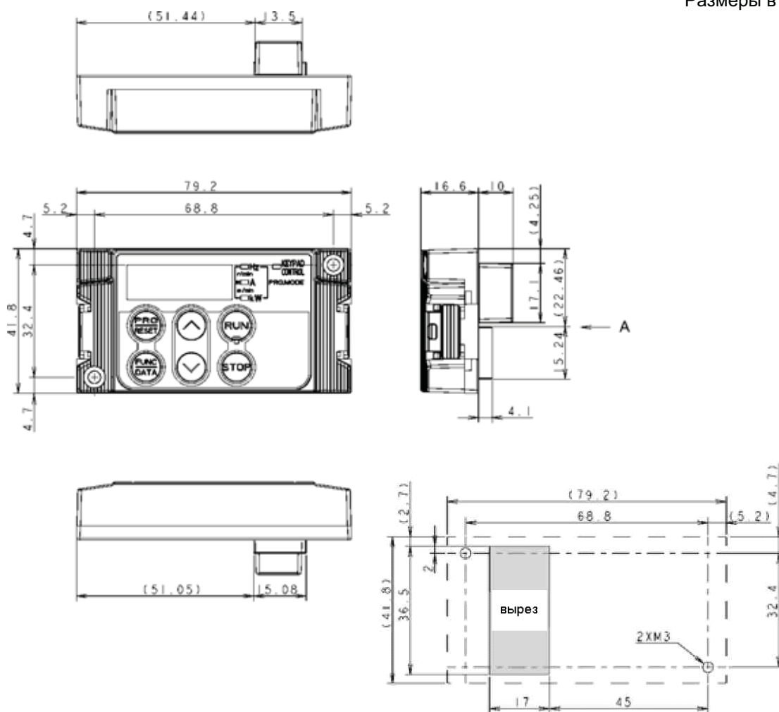
Размеры отверстий для монтажа панели
