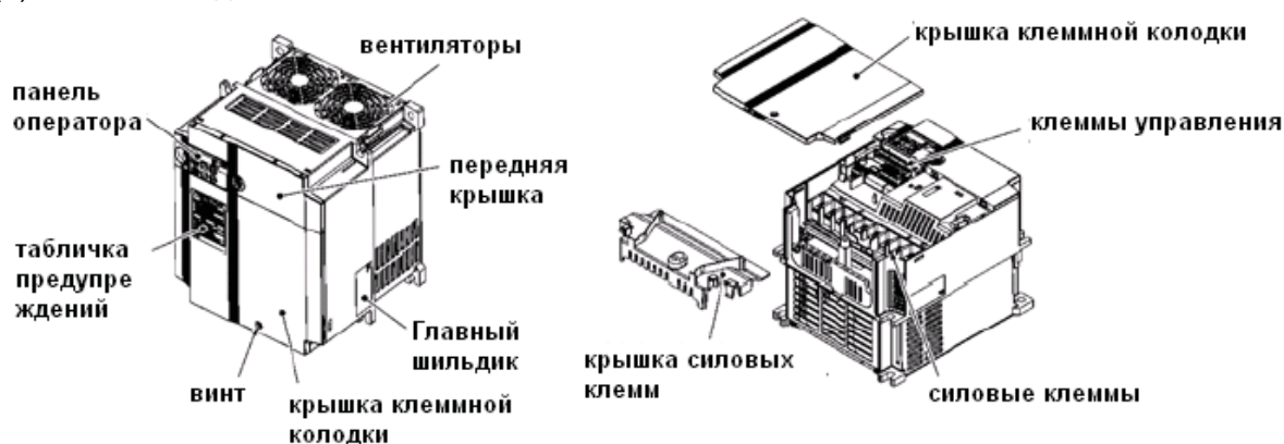
Рисунок 1.2 Внешний и внутренний вид ПЧ (FRN15E1S-4E)
