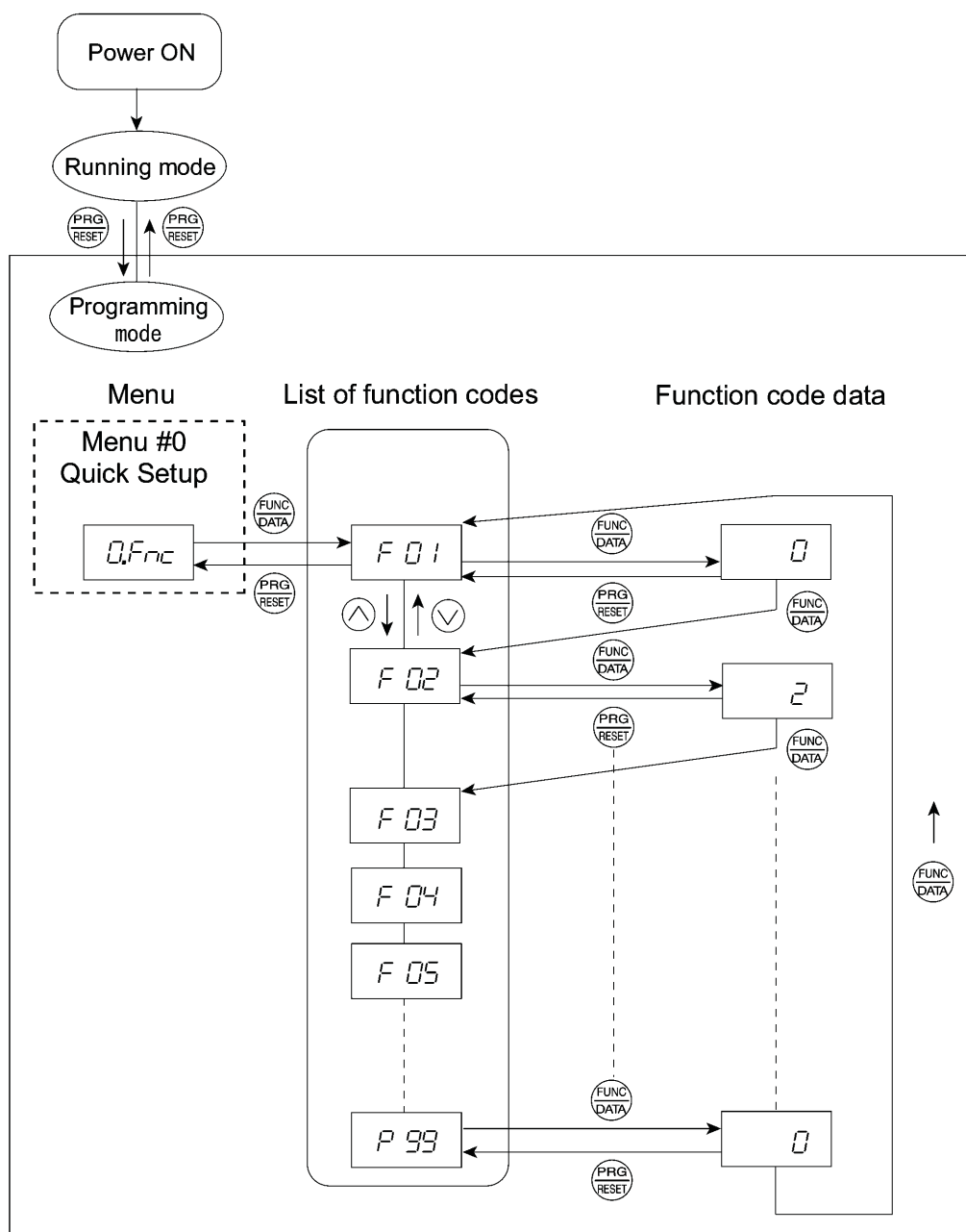
Рисунок 3.2 Переход меню в Меню #0 "Быстрая установка"
