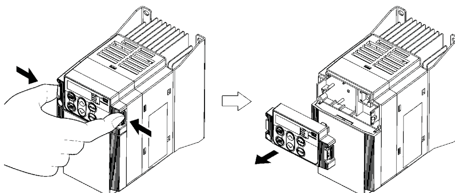
Рисунок 2.26 Снятие панели
