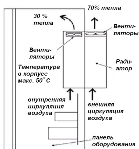
Рисунок 2.2 Внешнее охлаждение
