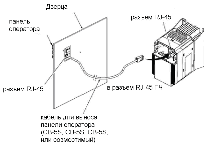
Рисунок 2.29 Подключения удлинительного кабеля
