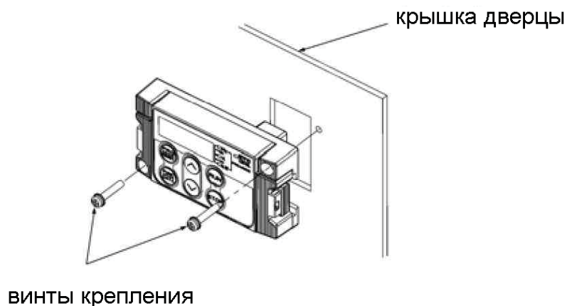
Рисунок 2.28 Установка панели на дверцу
