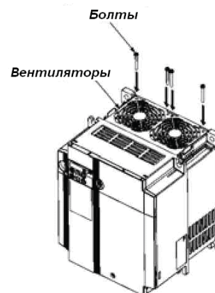
Рисунок 2.3 Крепление охлаждающих вентиляторов
