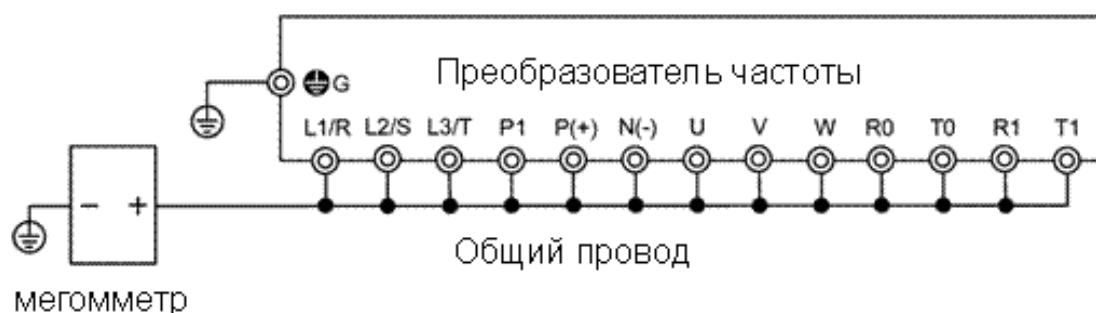
Рисунок 7.2 Измерение мегомметром
